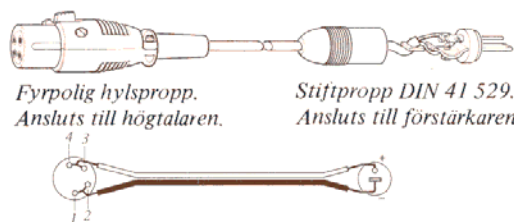
Bild 7 HÖGTALARKABELN
